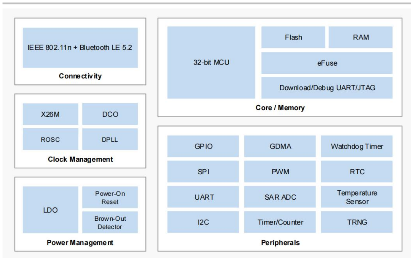
图 1：功能框图
