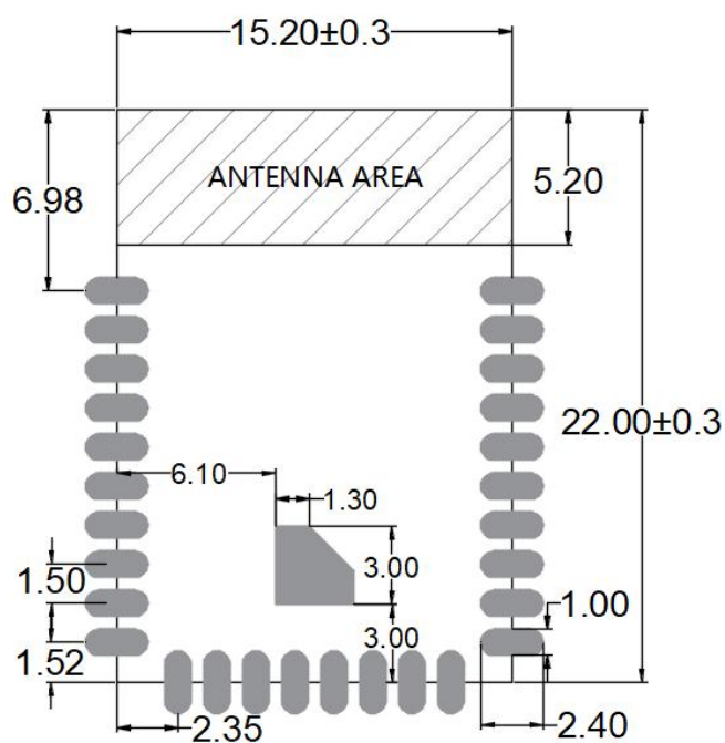
图 17: 建议封装尺寸图
