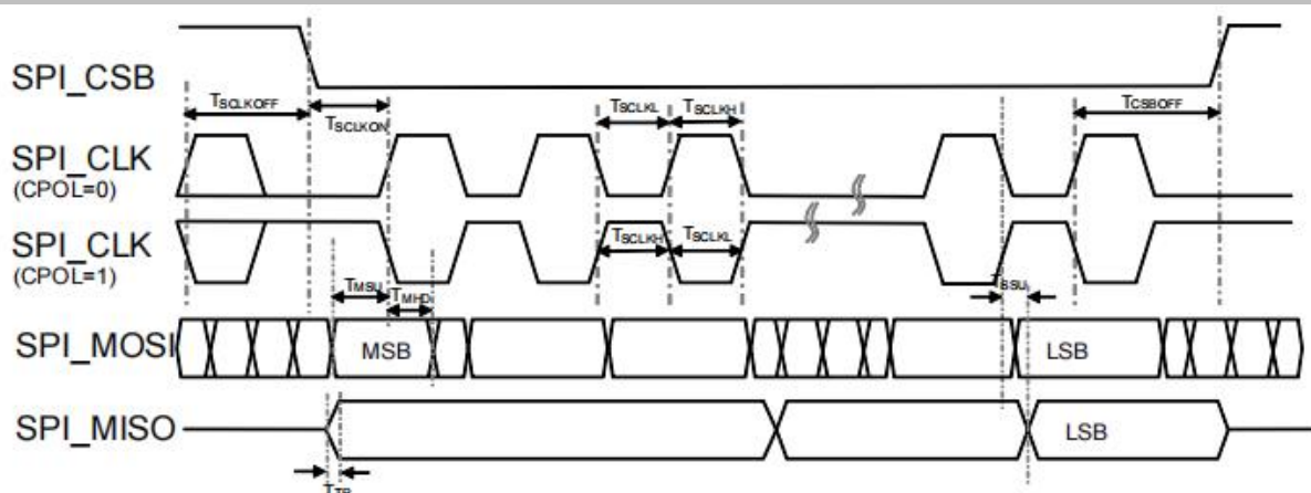
图 13: SPI 从机时序图
