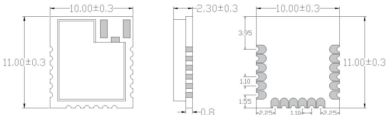
图 16: 模块俯视及侧视尺寸图
