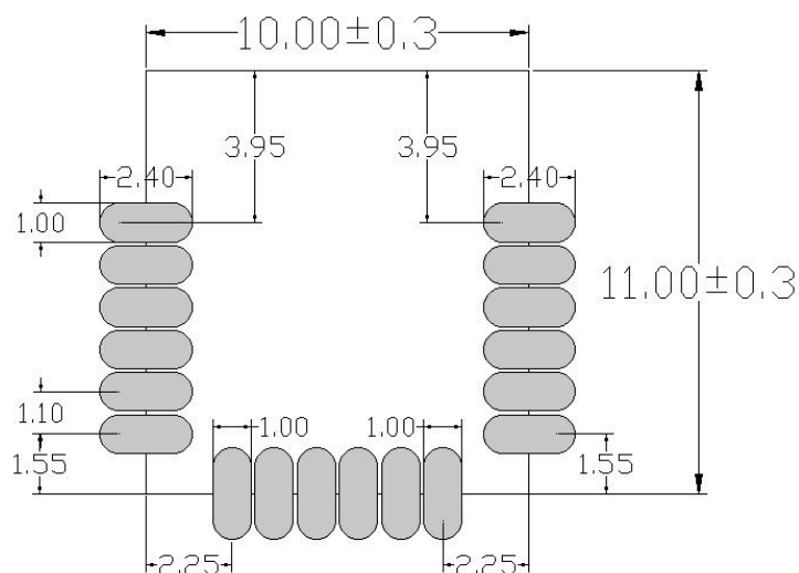
图 17: 建议封装尺寸图
