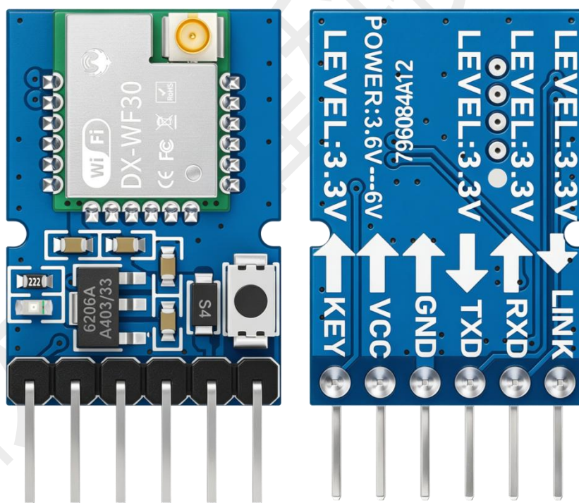
图 18: 模块俯视图和底视图
