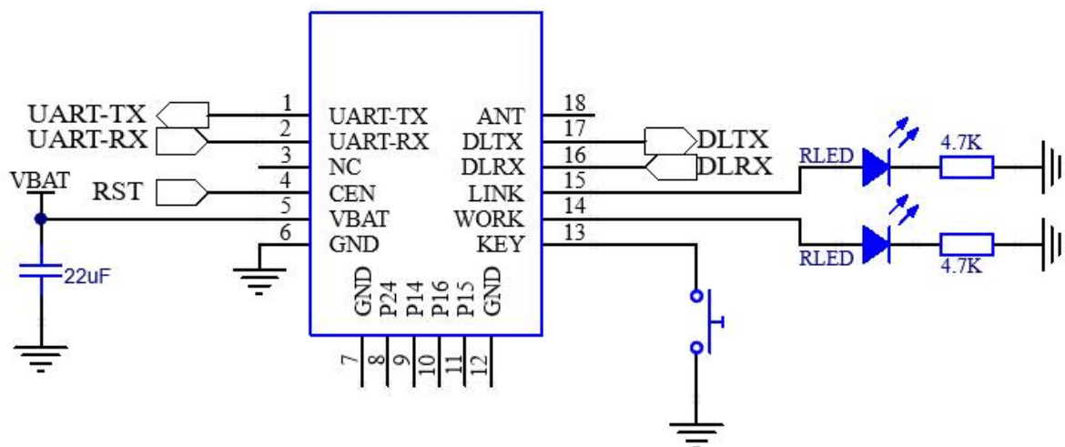
图 14: 典型应用电路
